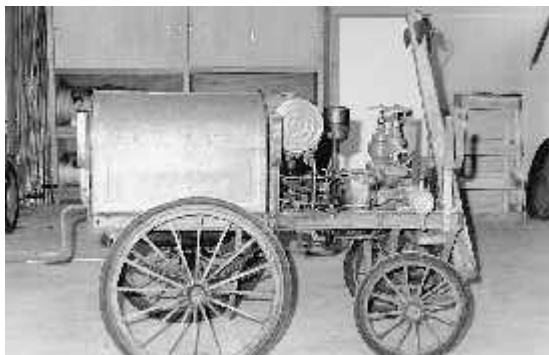
<手引ガソリンポンプ (昭和8年、北井号)>
